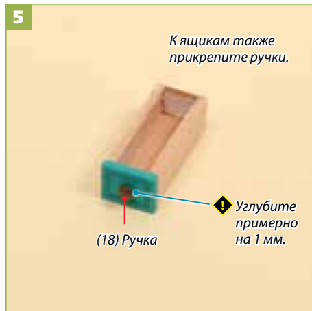
5 Так же небольшим количеством секундного клея прикрепите ручки в отверстиях в передней части ящиков.
