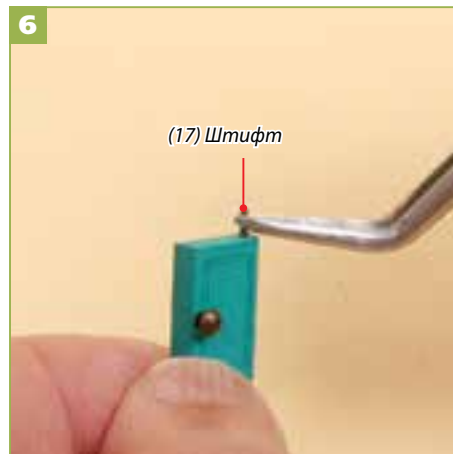
6 Вставьте штифт в отверстие в дверце.
