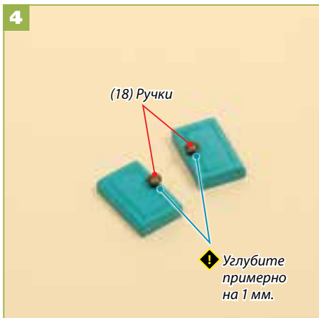
4 Секундным клеем закрепите ручки (18) в отверстиях дверец.
